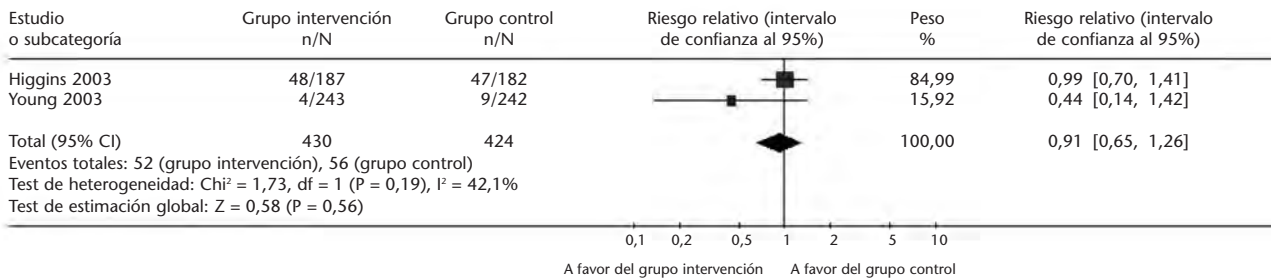
Figura 6. Metagráfico para la mortalidad específica. Grupo control DAI.
